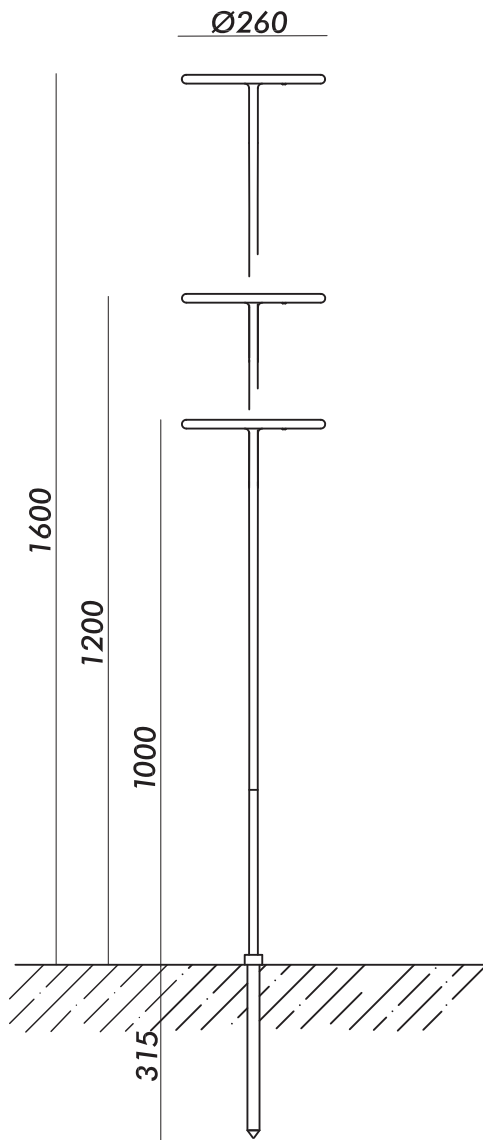
PUCK - 1190210
